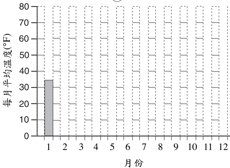
氣候分區 ⑤ 的每月平均溫度
