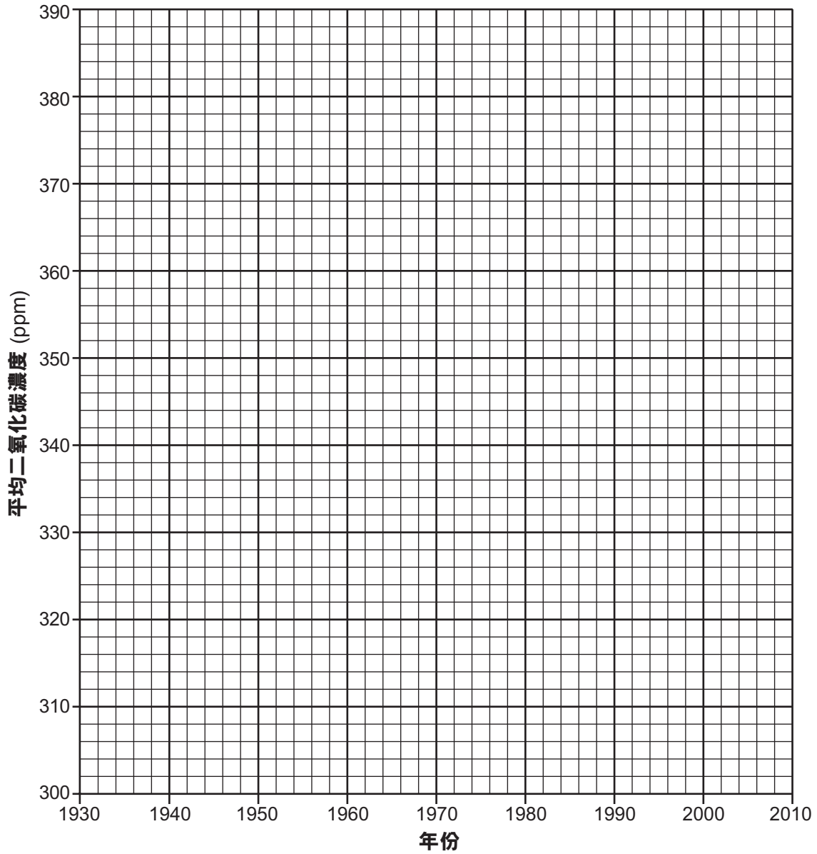
地球大氣中平均二氧化碳濃度
