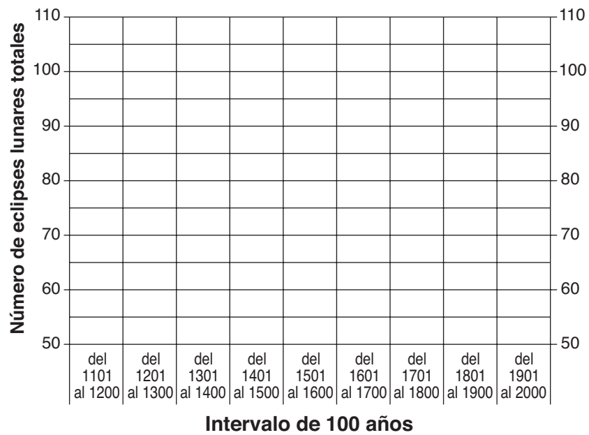
Eclipses lunares totales de cada siglo
