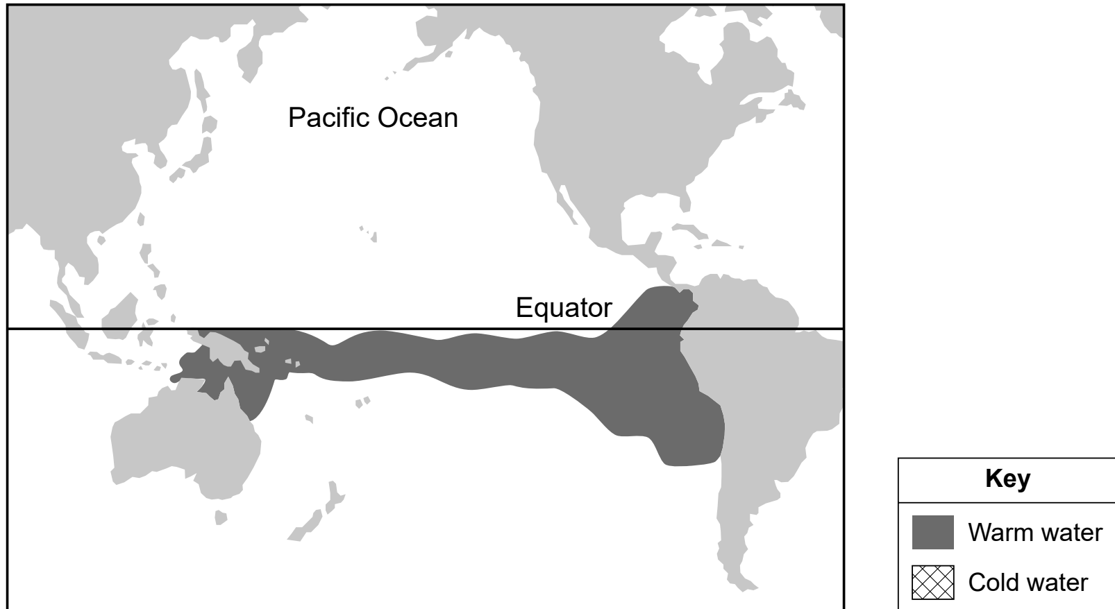
Map B: El Niño Conditions
