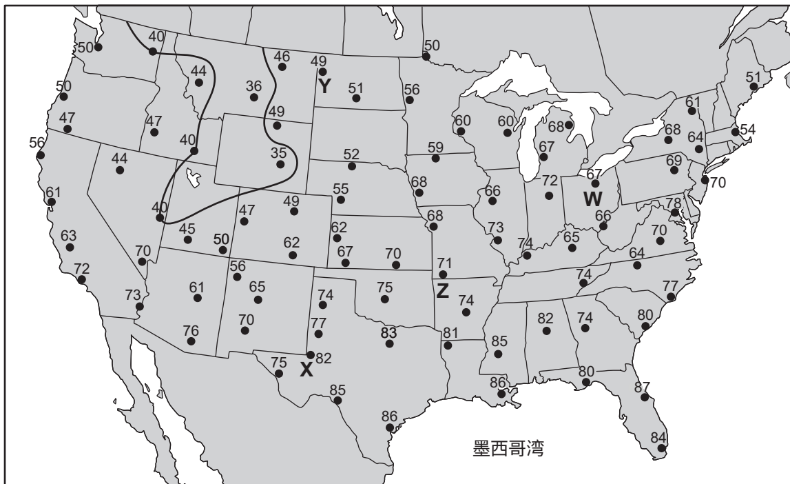
2010年10月25日地表空气温度(°F)
